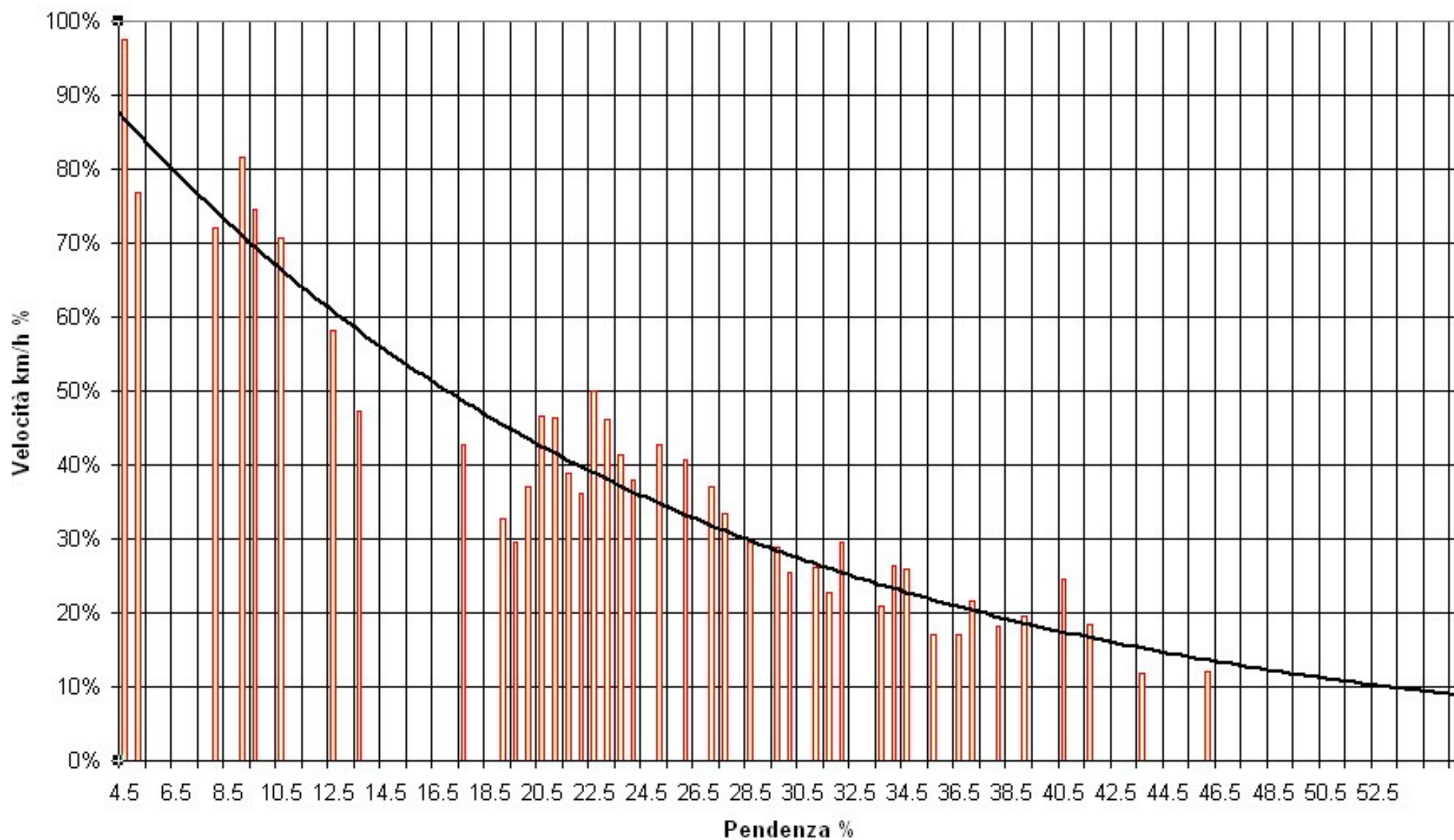
Velocità km/h % vs.Pendenza %
